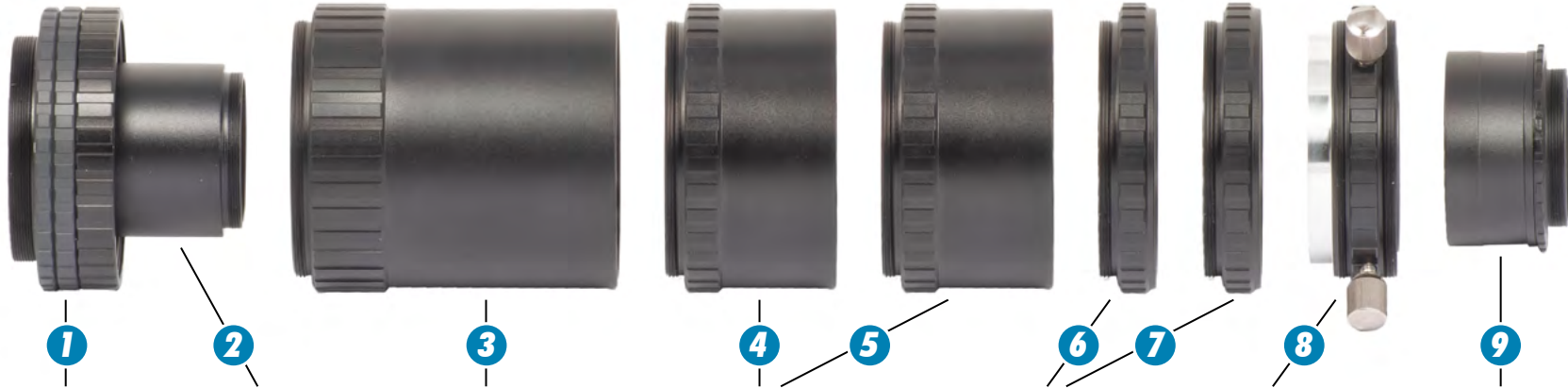
M68 Tele-Kompodium mit TZ-4 System
