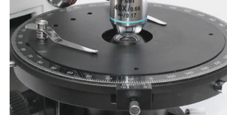
Platine à polarisation, centrable et rotatif
